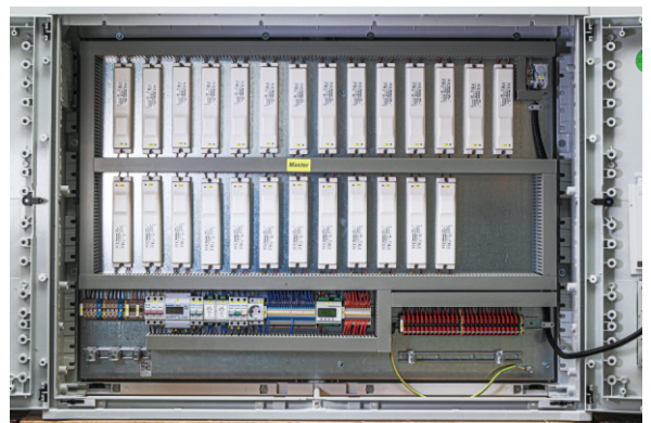
Converterschrank „Master“
