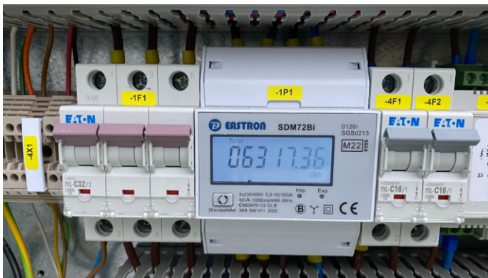
Energiezähler
