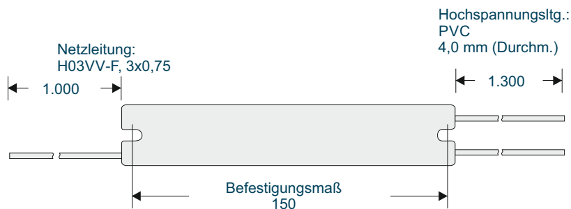
Gehäusefarbe: weiß Abmessungen in Millimeter
